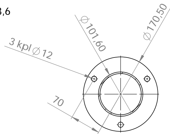
Leikkaus A-A Mitta 1:5
